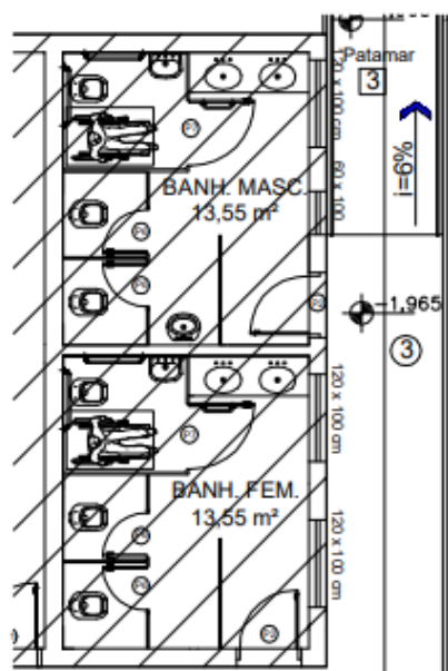
Figura 70 – Projeto de banheiro adaptado do Campus Avançado Carmo de Minas
